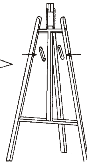
Bolt: 6mm×70mm×2pos
